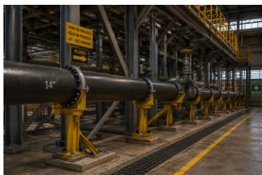
Tubulação
